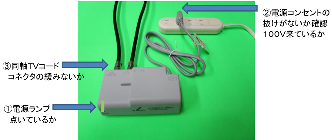
DXアンテナ V-ONU電源供給器(PS) このタイプのものが多く設置されている
